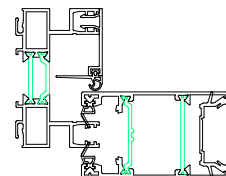
Capot latéral
